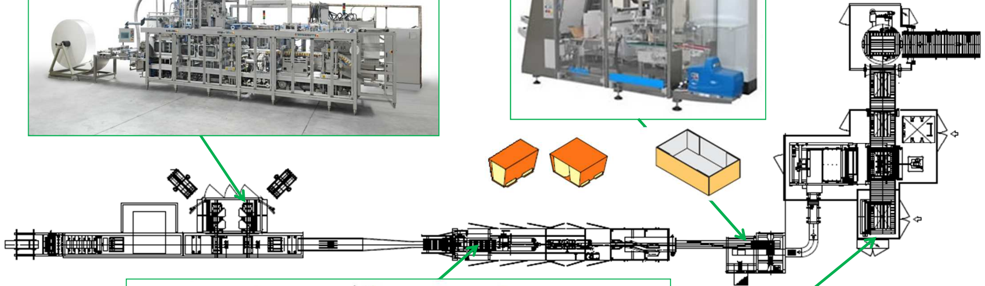
码垛机 Palletizer
